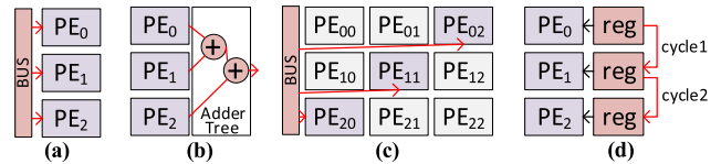
Fig. 5. Spatial reuse functions: (a) broadcast; (b) reduction; (c) diagonal; (d) shift.
